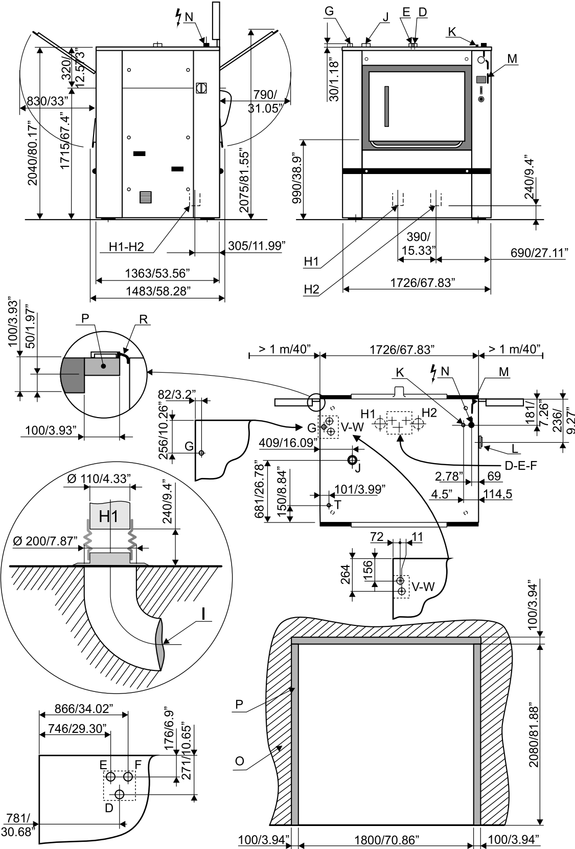
Barriereversion WB6 90: Zeichnung 07100159
